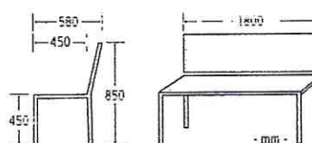
Ławka URBIS
